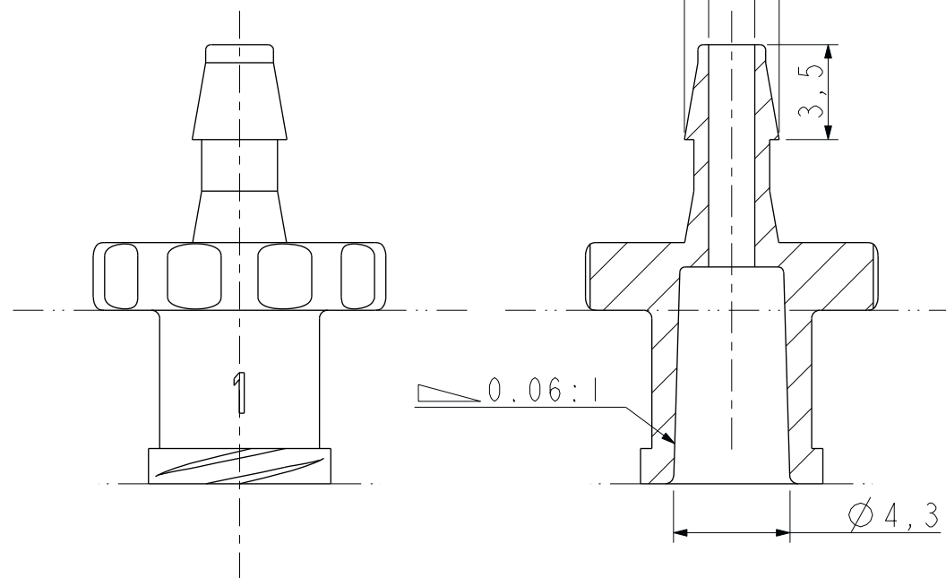
截面 A-A
