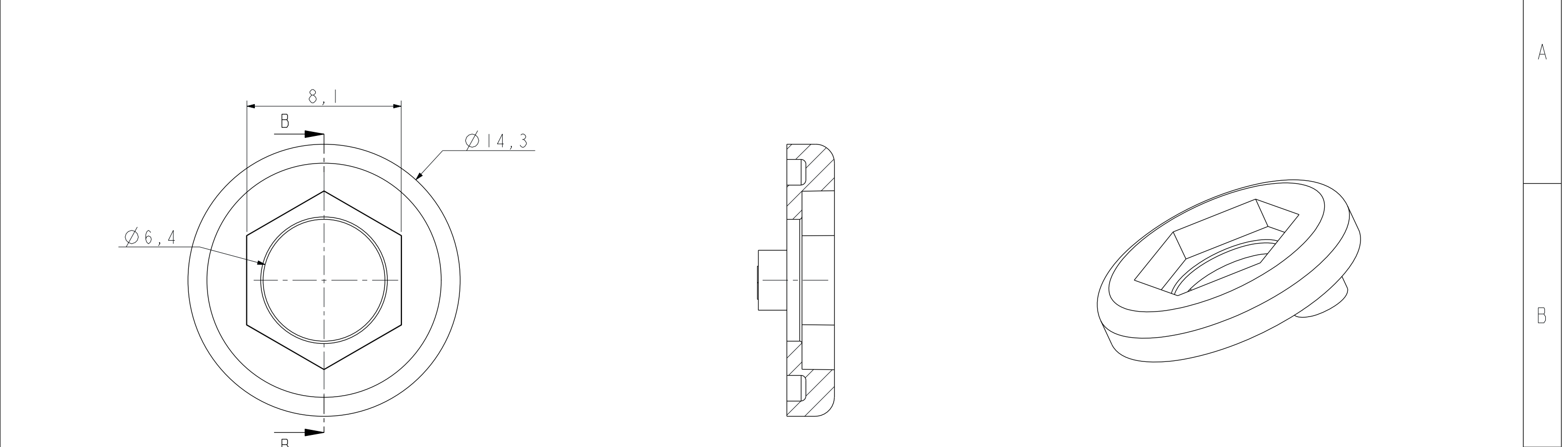
截面 B-B
